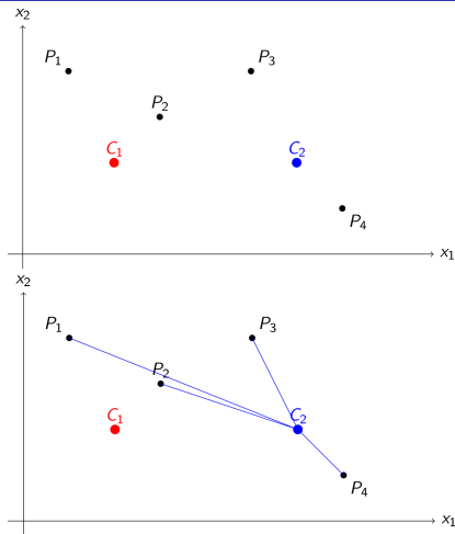
Figura: Funcionamento do algoritmo K-Means.
